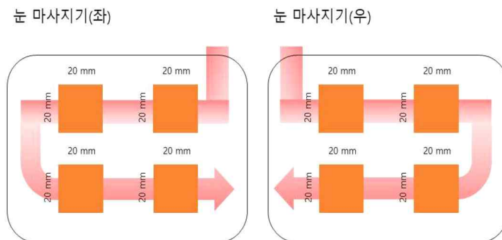
[그림A.1] 눈마사지기온도측정위치
